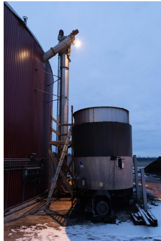
Kuivalanta syötetään ensimmäiseen reaktoriin apevaunun ja ruuvikuljettimien avulla
